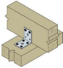
Winkelverbinder Stahl sendzimirverzinkt ohne Rippe
