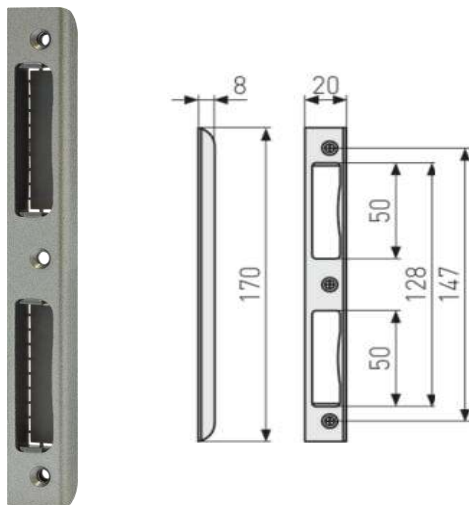
Schließblech für Innen- und Korridortüren " WSB 170 " Stahl - Schließblech mit Kunststoffeinlage silberfarbig
