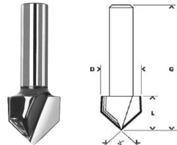
Bosch V-Nutfräser "Standard for Wood" mit hoher Schneidleistung für das Schneiden feiner Schriftzüge
