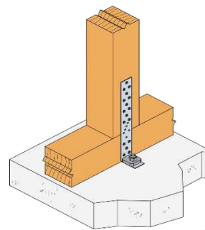
AH Zuganker als Zugverbindung von Holzbauteilen an Beton.
