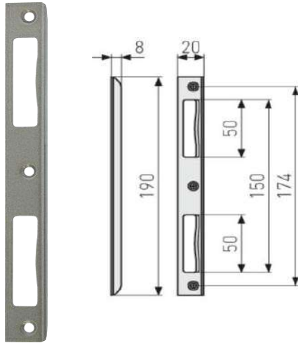
Schließblech für Haustüren " WSBHT190 " Stahl - Schließblech Hammerschlag gold
