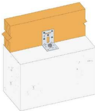
Winkelverbinder mit beidseitigem Langlöchern bietet eine vielfältige Montageausgleichsmöglichkeit inkl. einer Rippenverstärkung
