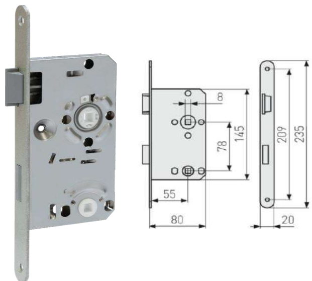
Einsteckschloss " ES WC " für Bad/WC Dornmaß: 55mm x Entfernung: 78mm Stulp 20 x 235 mm rund silber Riegel und Falle aus Kunststoff
