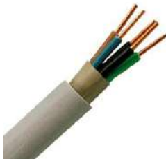
Feuchtraumkabel "NYM-J 5x2,5 mm 2 in verschiedenen Rollenlängen
