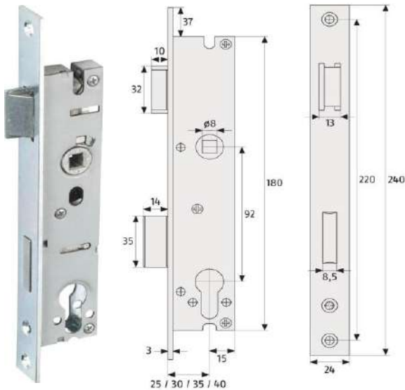
Rohrrahmenschloss " ESR PZ " Dornmaß: 25-40mm x Entfernung: 92mm Stulp 24mm kantig verzinkt - für Profilzylinder Riegel und Falle aus Metall
