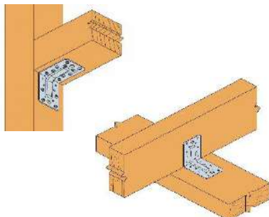
Winkelverbinder Stahl sendzimirverzinkt mit Rippe
