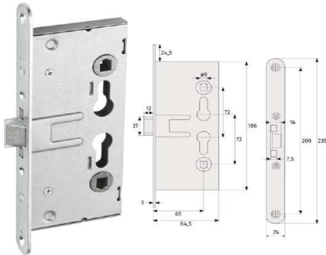
Einsteckschloss " EFS 65 " für Feuerschutztüren Dornmaß: 65mm x Entfernung: 72mm Stulp 24mm rund - für Profilzylinder Riegel und Falle aus Metall
