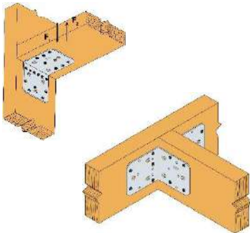
Winkelverbinder Stahl sendzimirverzinkt ohne Rippe
