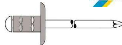
GESIPA Blindnieten PolyGrip® mit Großkopf Hohlriet: Aluminium-Legierung - Nietdorn: Stahl, verzinkt Großer Klemmbereich mit nur einem Blindniete
