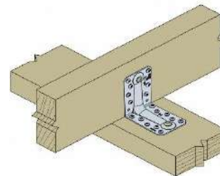
Winkelverbinder mit Rippe Edelstahl (V4A) 1.4401 bzw. 1.4404 gemäß EN10088
