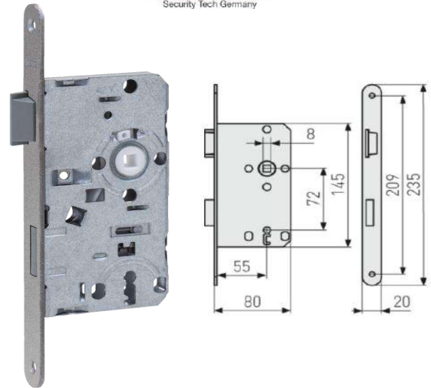
Einsteckschloss " ES BB R " für Zimmertüren Dornmaß: 55mm x Entfernung: 72mm Stulp 20 x 235 mm rund silber - für Bundbartschlüssel Riegel und Falle aus Kunststoff
