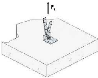
Winkelverbinder mit einseitigem Langloch, bietet eine Montageausgleichsmöglichkeit inkl. einer Rippenverstärkung
