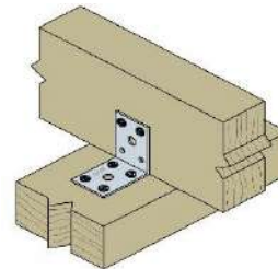
Winkelverbinder Edelstahl (V4A) 1.4401 bzw. 1.4404 gemäß EN10088
