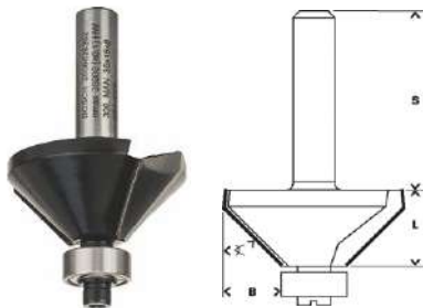
Bosch Fasefräser 45 Grad "Standard for Wood" zweischneidig mit Anlaufkugellager und mit hoher Lebensdauer für gleichmäßiges und splitterfreies Fasen
